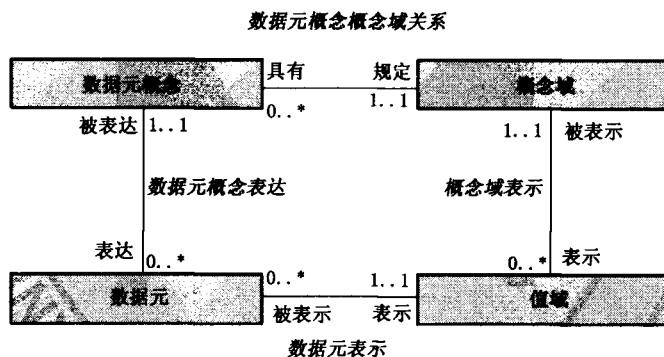
图 3 高层元模型
